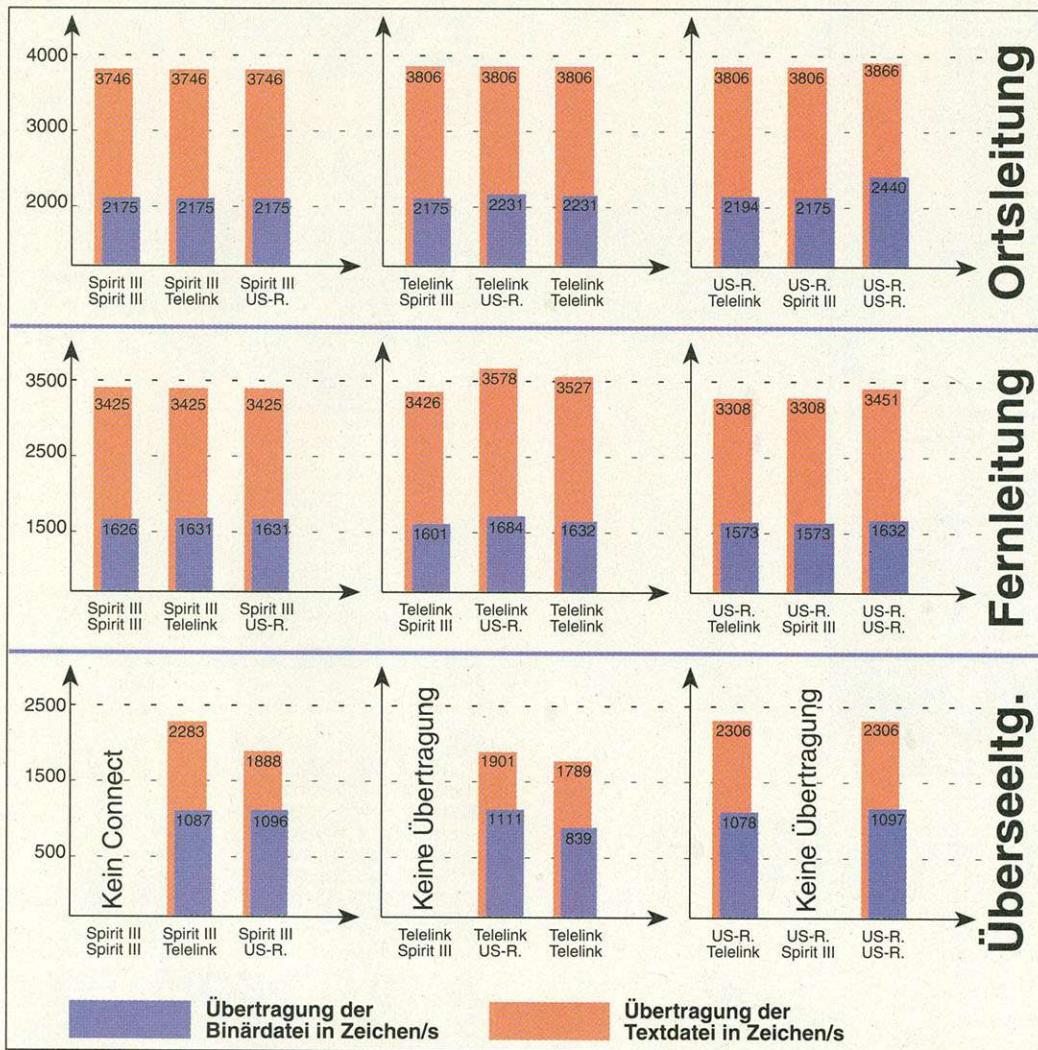
Auf einen Blick: Die Balkendiagramme spiegeln alle Testergebnisse wider – die der Orts-, Fern- und Überseeltg. Die bei einer Ortsleitung erzielten Werte sprechen für sich.
